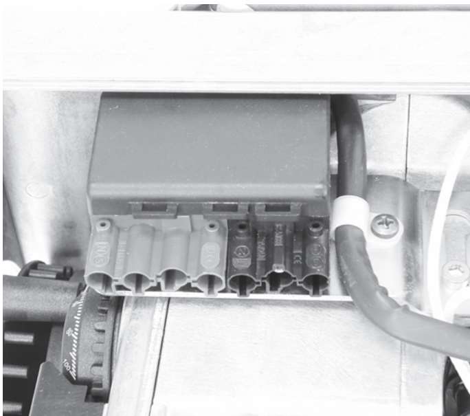
Abbildung 32 - Netzanschluß - Eurostecker Figure 32 - Power connection - Euro-plug - Prise Euro du raccordement sur secteur
