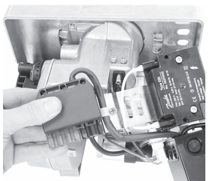
Abbildung 29 - Steuereinheit abgenommen Figure 29 - Control unit removed - Organe de commande retiré
