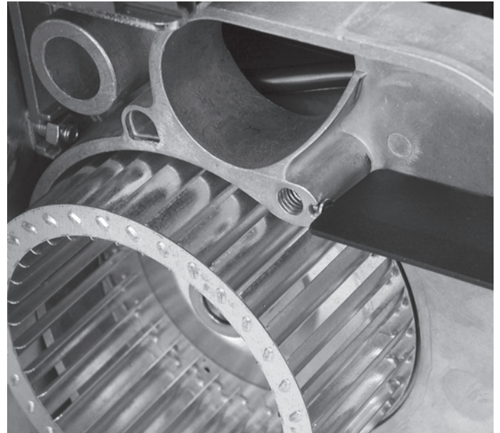
Abbildung 27 - Einbaulage der Luftklappe Figure 27 - Installation position of the air flap - Position de montage du clapet d'air
