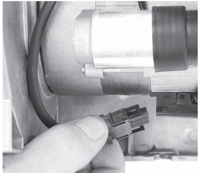
Abbildung 34 - Steckanschluß für Motor Figure 34 - Plug connection for motor - Prise de raccordement pour le moteur
