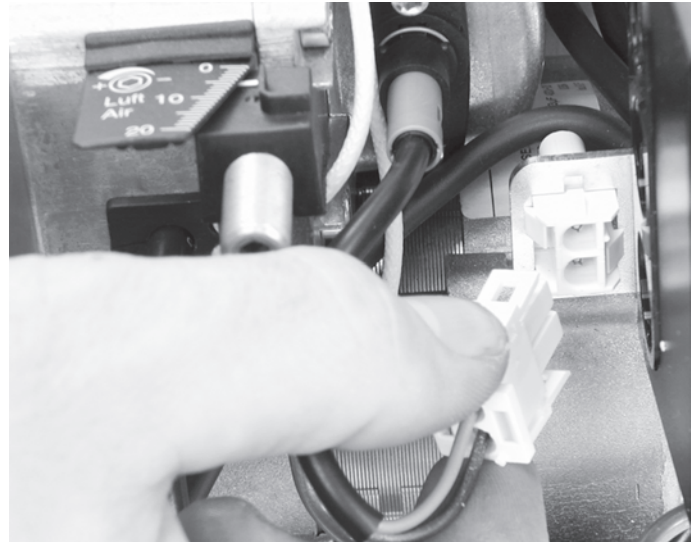
Abbildung 33 - Steckanschluß für Fotowiderstand Figure 33 - Plug connection for photo resistor - Prise de raccordement pour la résistance photo-électrique
